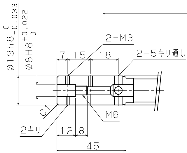
< A 詳細図 >
